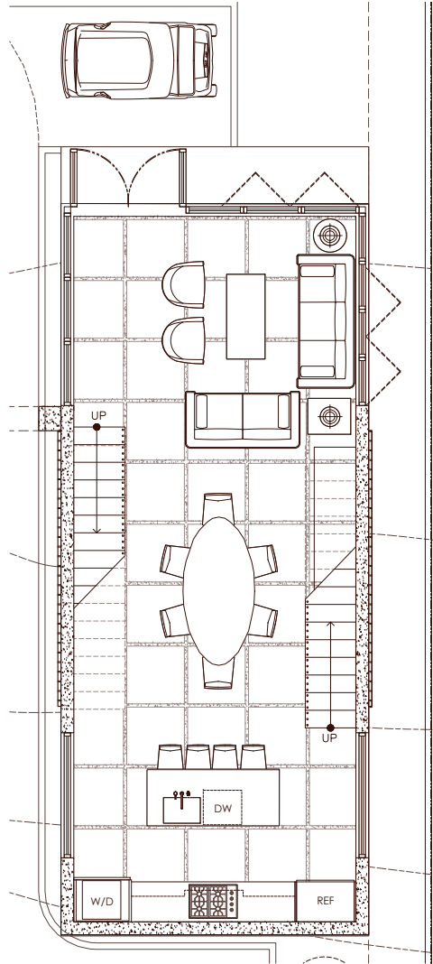
① CASITA 4 LEVEL 1 FLOOR PLAN SCALE: 3/8" = 1'-0"
