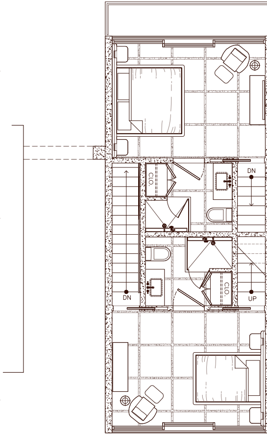
② CASITA LEVEL 2 FLOOR PLAN SCALE: 3/8" = 1'-0"
